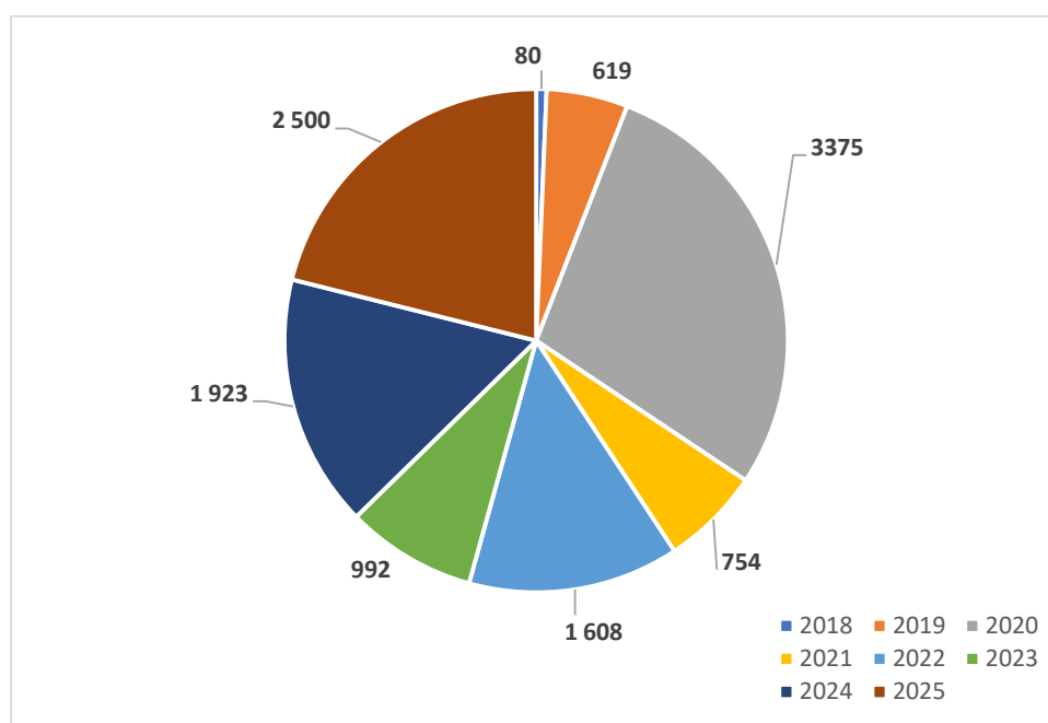
Figure 3 : Linéaire de réseaux AEP renouvelés depuis 2018
