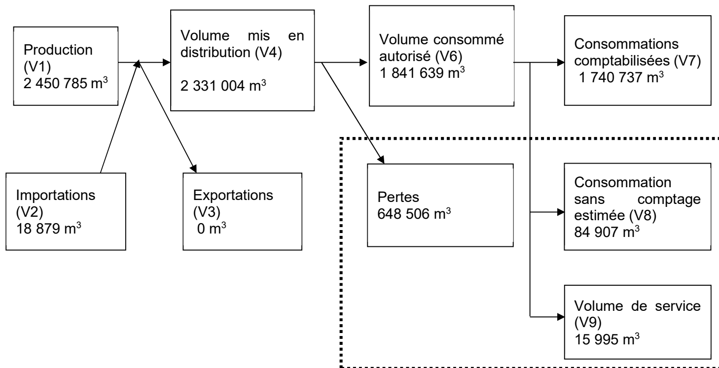
Figure 9 : Bilan des volumes 2025
