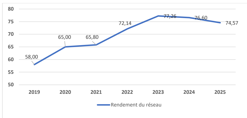
Figure 12 : Evolution du rendement de réseau
